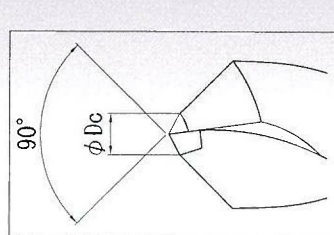
刃先拡大図
